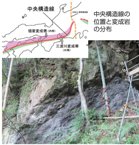
中央構造線長篠露頭
