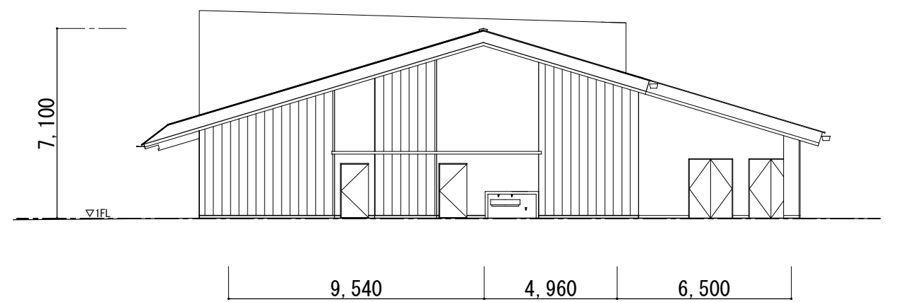
東面立面图
