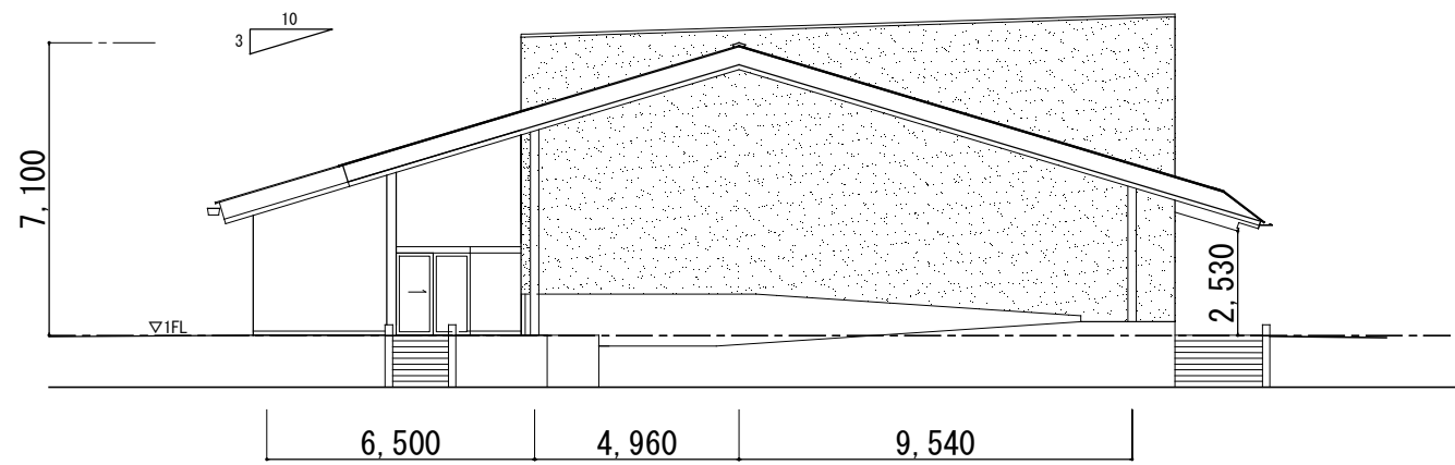
西面立面图
