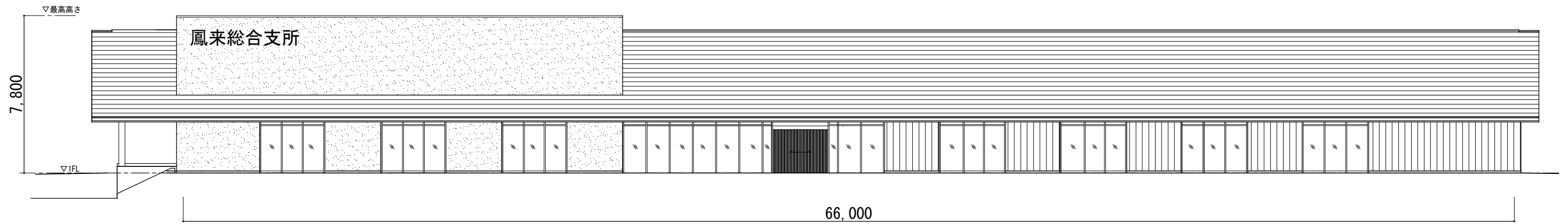
南面立面图
